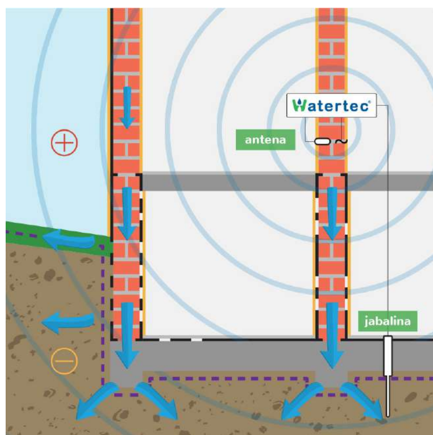
Sistema Watertec® en funcionamiento.
